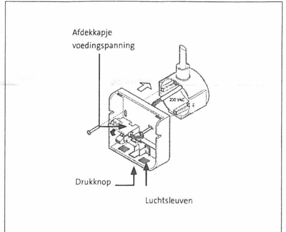
Fig. 2 - Montage wandframe
